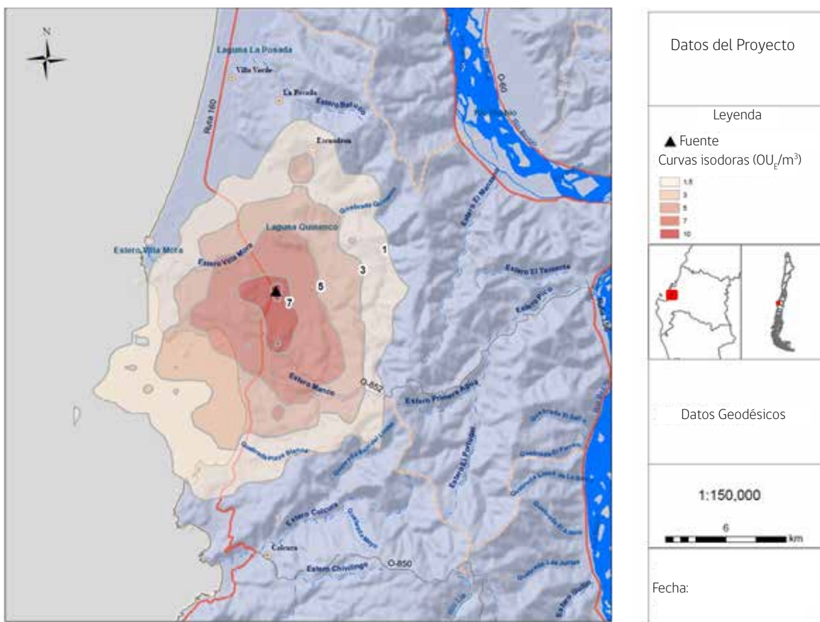
FIGURA 10. Mapa de curvas isodoras
