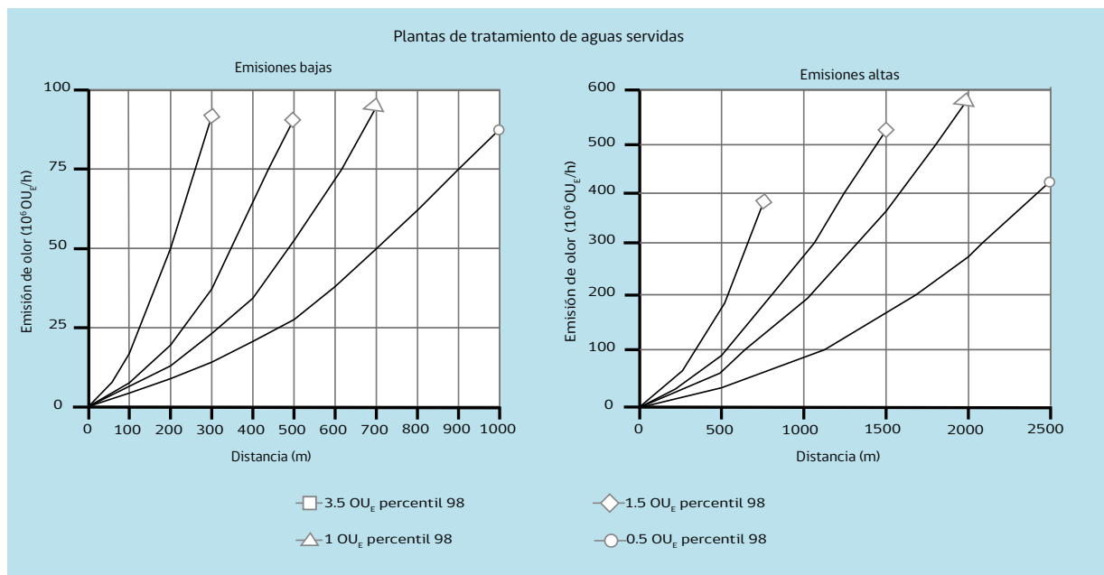
FIGURA 9. Nomogramas para plantas de tratamiento de aguas servidas: concentración de olor en inmisión
